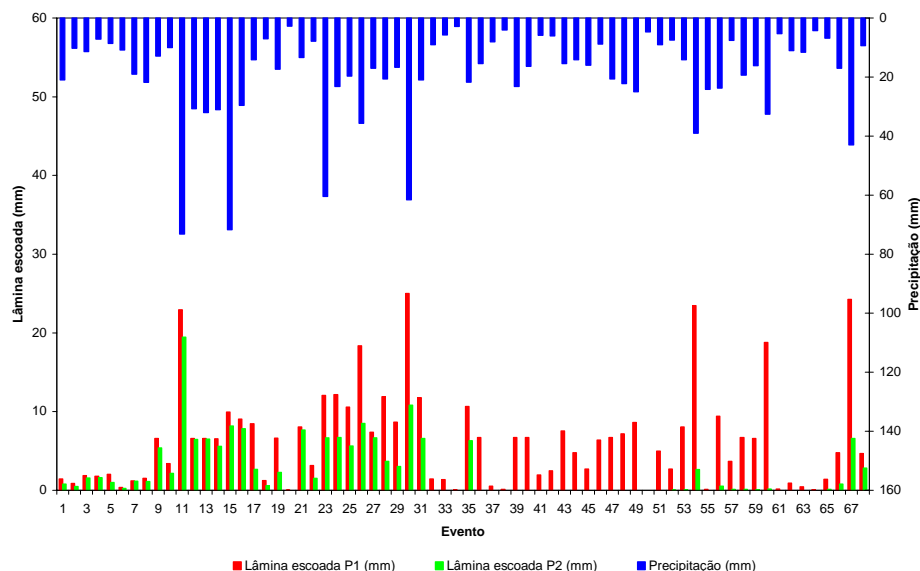
Figura 2. Lâmina escoada em função da precipitação no período considerado.
