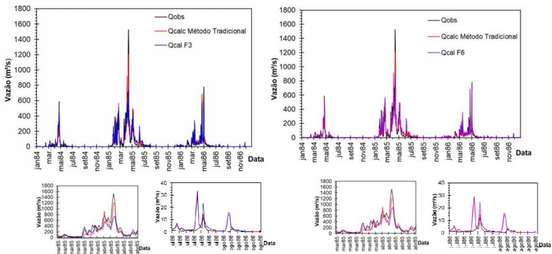
Figura 4. Comparação entre hidrogramas observados e calculados (F3) e (F6) em parte do período de calibração.
